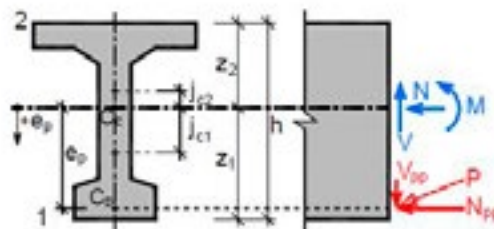
Obr. 1 Předpjatý průřez, účinky zatížení a předpětí
